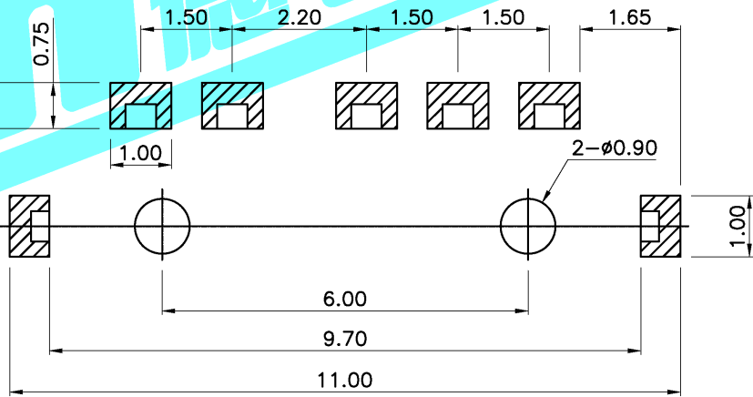
P.C.B Layout
